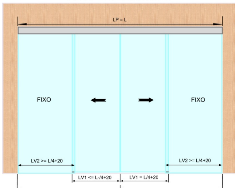
PORTA - 2 FOLHAS + 2 FIXOS
