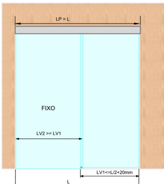
PORTA - 1 FOLHA + 1 FIXO
