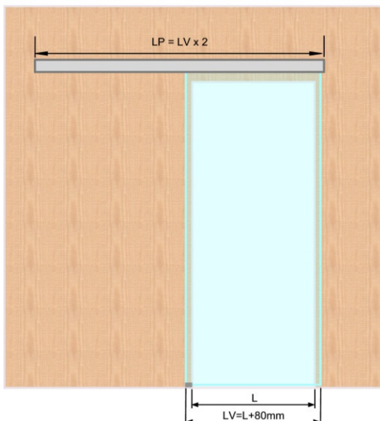
PORTA ÚNICA - 1 FOLHA
