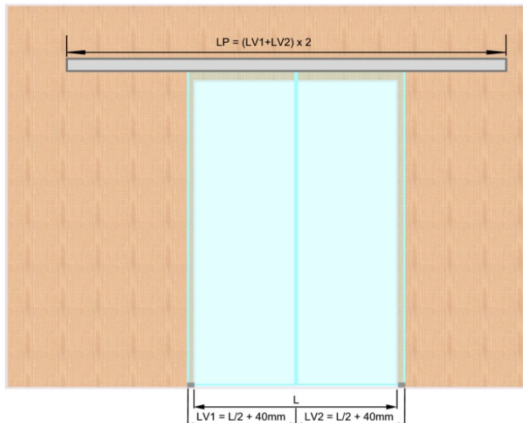
PORTA - 2 FOLHAS
